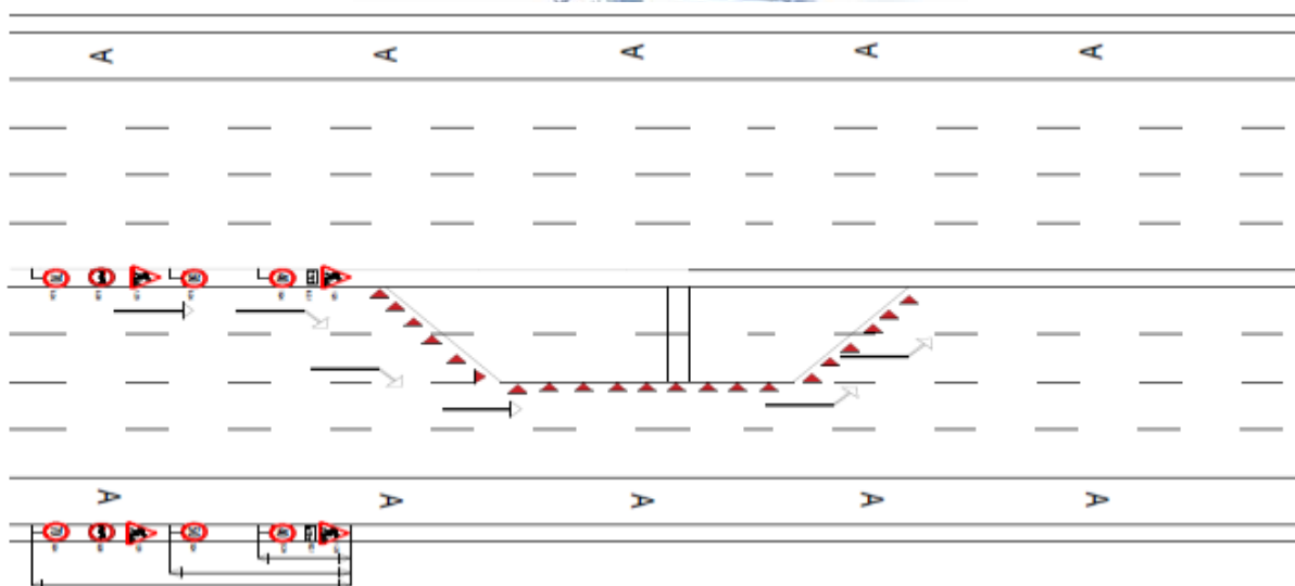
2-rasm. Besh tasmali yo‘lning chapdan 2ta tasmasi mirlanayotgan yo‘l bo‘lagida harakat xavfsizligini ta‘minlash va ta‘mirlanayotgan yo‘l bo‘lagini yo‘l to‘siqlari bilan to‘shish sxemasi.
